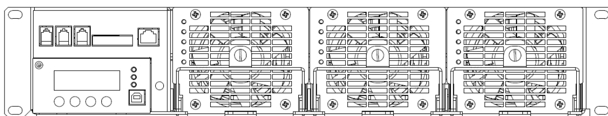
Рисунок 2.2 – Модульный каркас Штиль PS2020KM с инверторами Штиль PS220/2000K, ver.2.1 (PS220/2000K (I), ver.2.1)
